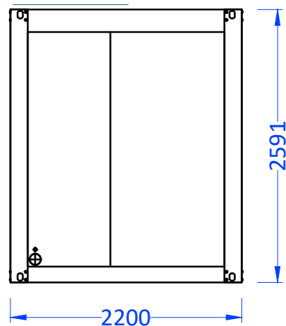
Ansicht "F"
