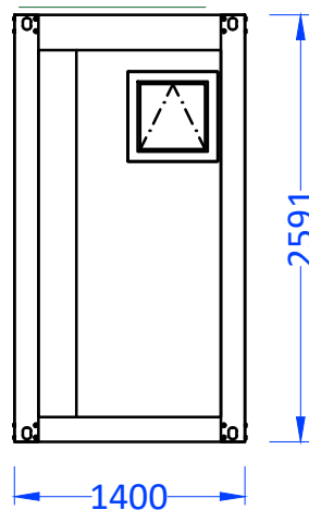
Ansicht "D"
