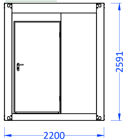
Ansicht "A"
