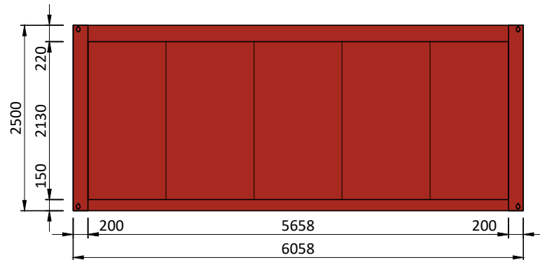
Ansicht "A"
