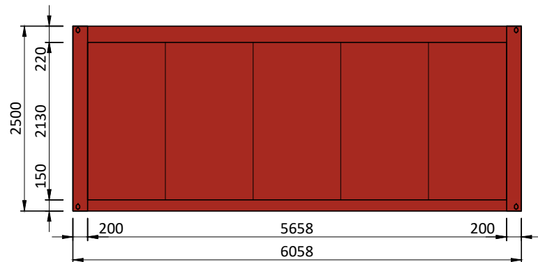
Ansicht "C"
