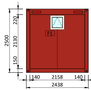
Ansicht "D"
