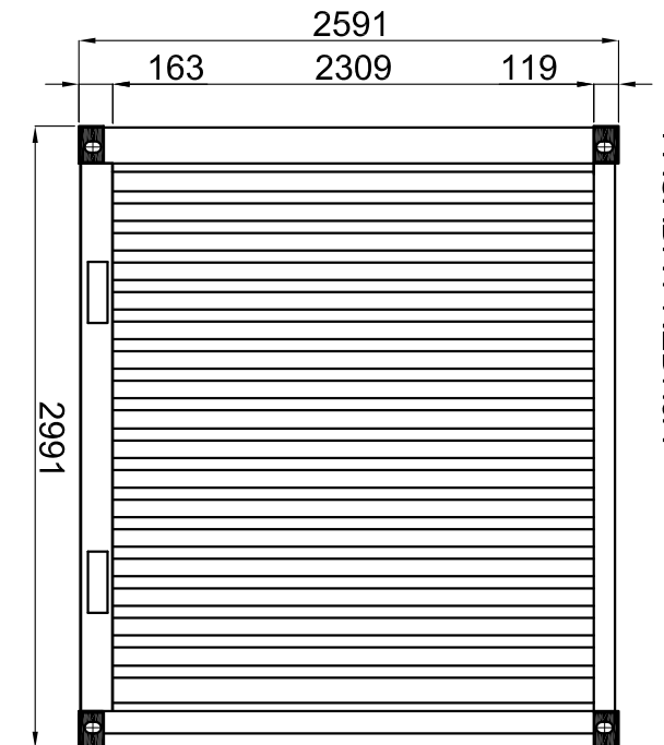
FASADA PREDNJA
