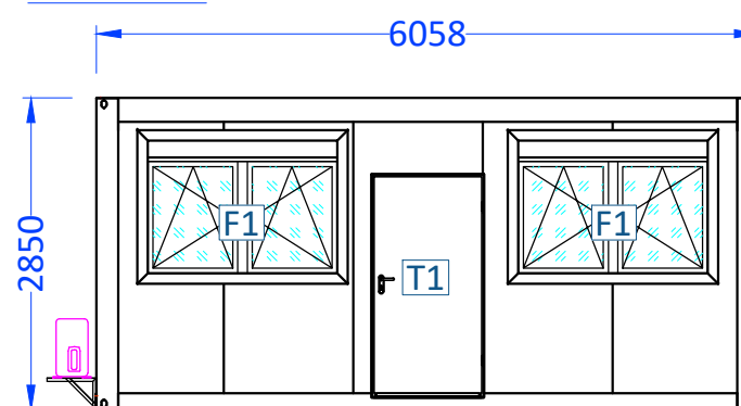
Ansicht "A"
